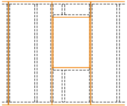
Fensteröffnung bei vertikalem Beplankungsstoß ohne Fugenversatz
