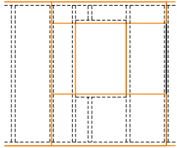
Fensteröffnung bei horizontalem Beplankungsstoß
