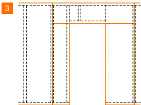
Türöffnung bei horizontalem Beplankungsstoß
