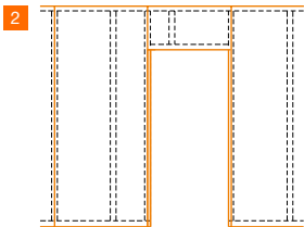
Türöffnung bei vertikalem Beplankungsstoß ohne Fugenversatz
